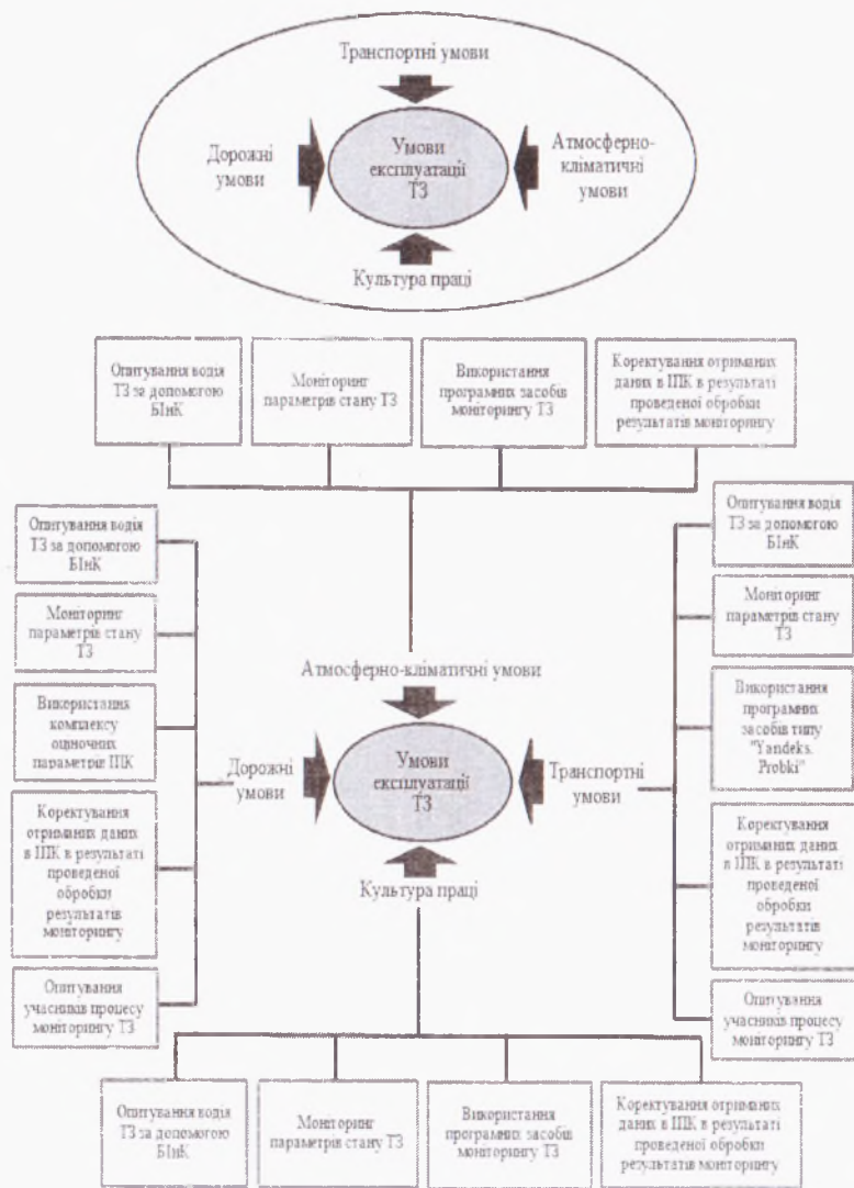
Загальна схема способів отримання і формування інформації про стан і умови експлуатації ТЗ в умовах ITS
